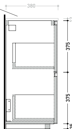
sezione longitudinale / section
