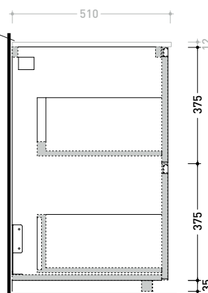
sezione longitudinale / section
