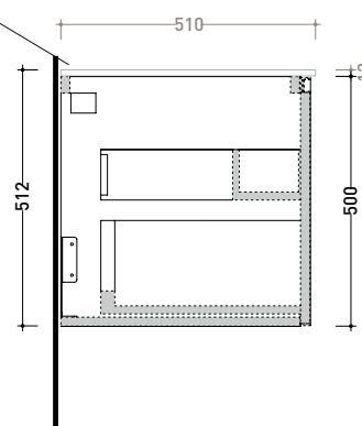
sezione longitudinale / section
