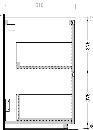
sezione
