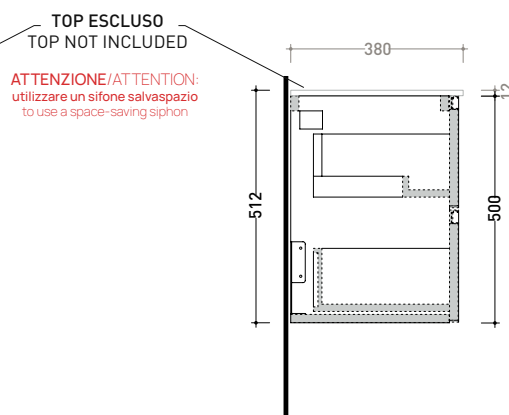
sezione longitudinale / section
