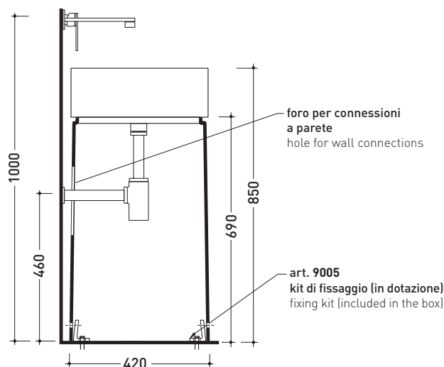
sezione longitudinale / section
