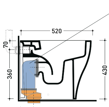
da/ from 100 a/ to 120 mm sezione longitudinale / section
