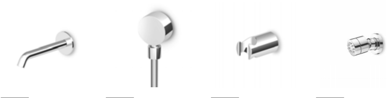
Z92183 Bocca di erogazione Wall spout Caño Z9380P Presa acqua Wall elbow Racor mural Z93781 Appendidoccia Handshower support Soporte ducha Z92896 Soffione laterale a getto fisso Lateral shower head with simple jet Rociador lateral con chorro fijo
