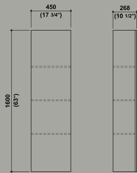
Morphing/unit colonna sospesa con anta wall unit
